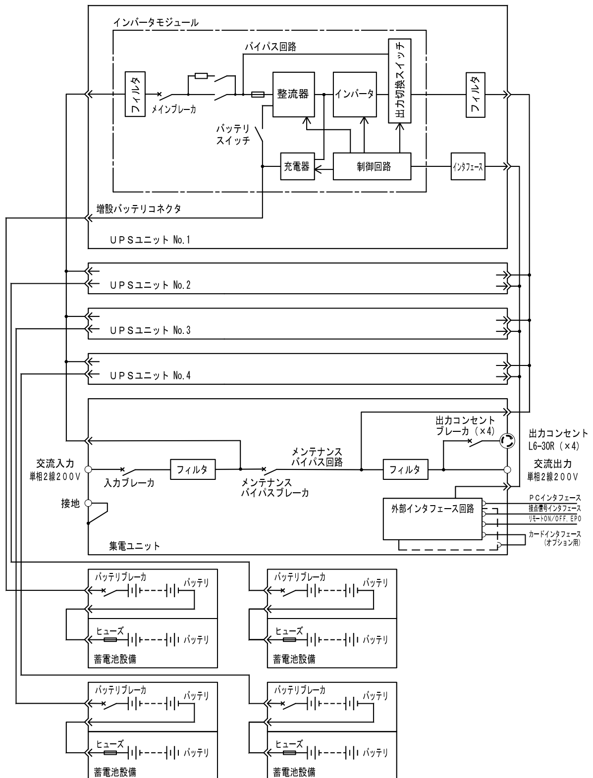
上図はFU-MS20-S2S2の回路系統図です。 バックアップ時間の仕様により蓄電池盤（バッテリー）の構成が異なります。
